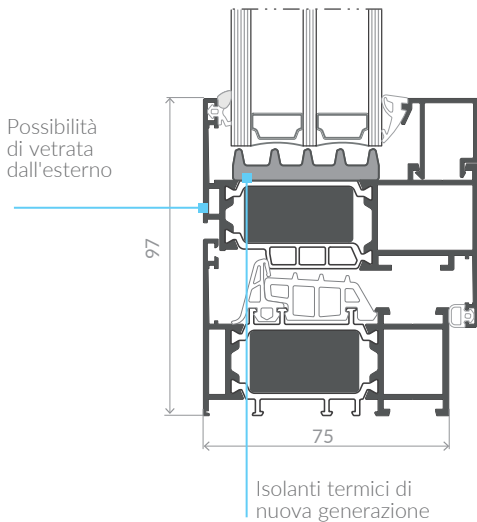
AS75 OKNO sezione finestra apribile
