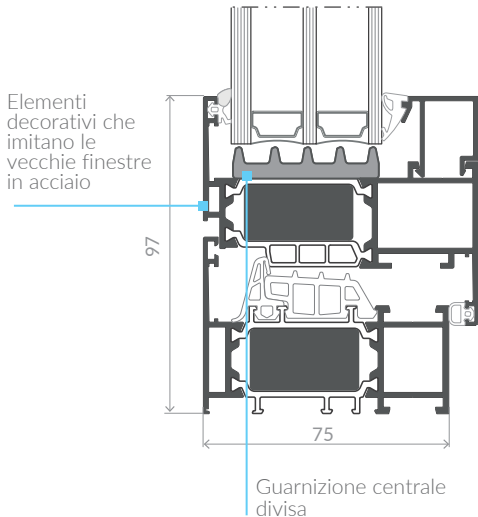
AS75 sezione tipo finestra INDUSTRIAL
