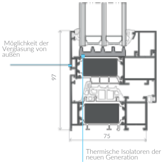
AS75 OKNO FENSTER Querschnitt durch ein Fenster
