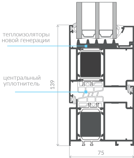
AS75 DRZWI ДВЕРИ Разрез через двери открываемые наружу
