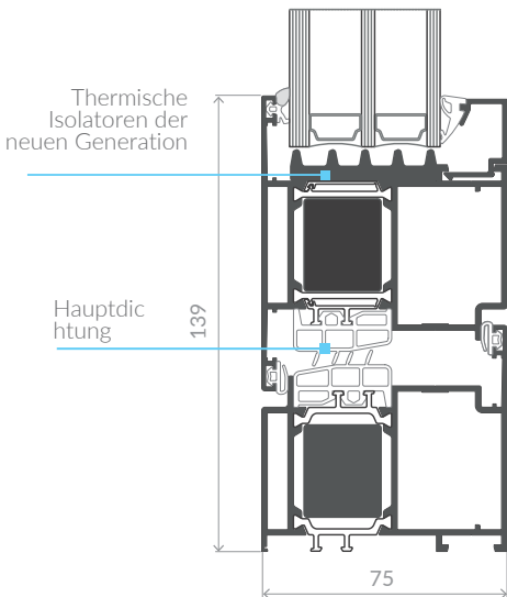
AS75 DRZWI TÜREN Querschnitt durch nach außen öffnende Tür
