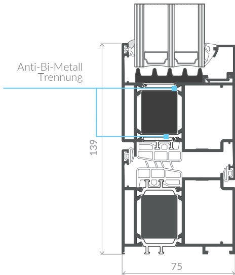
AS75 DRZWI TÜREN Querschnitt durch nach innen öffnende Tür
