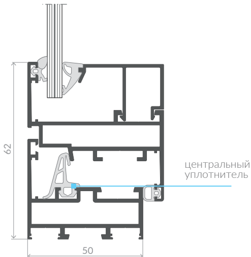
ACS 50 Разрез через открываемое окно
