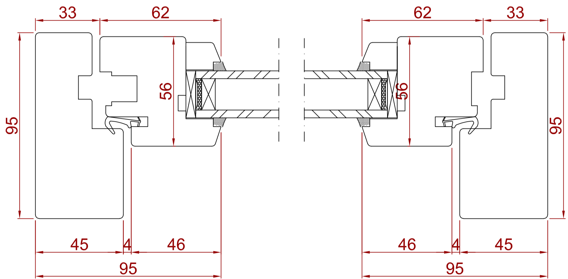
PRZEKRÓJ A
