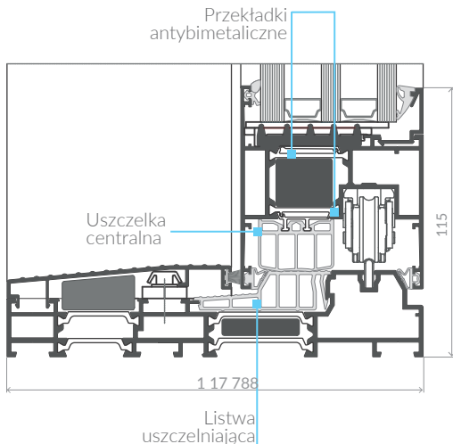
AS178HS PRO SLIM Przekrój przez drzwi przesuwne na poziomie posadzki
